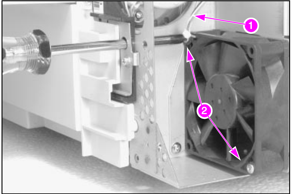
Fan 2, LVPS
