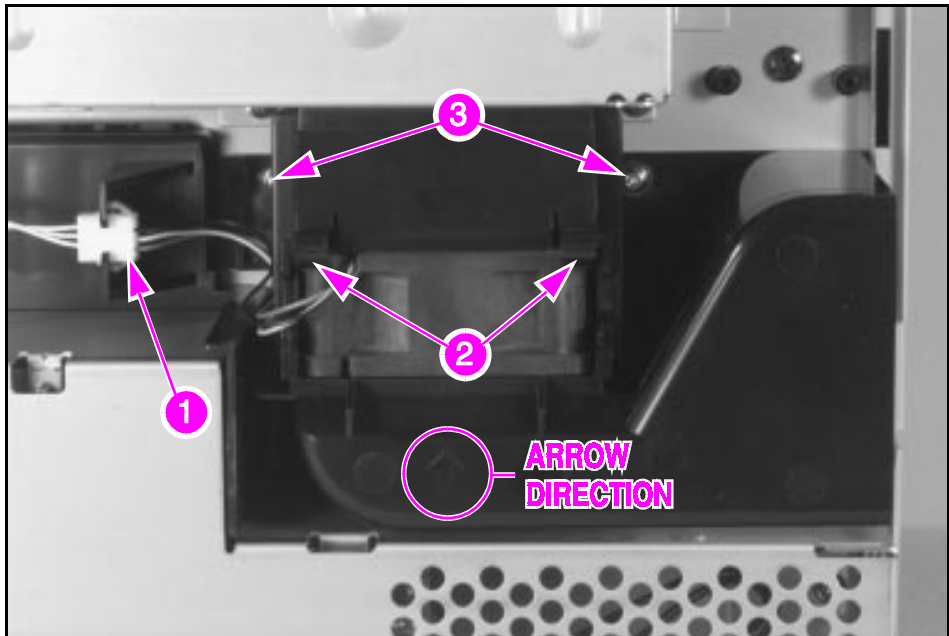
Fan 3, Formatter
